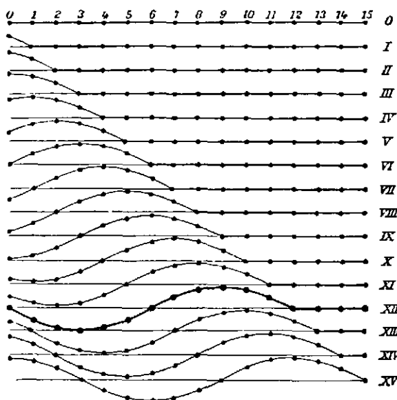
ציור 8 התהוותו והתקדמותו של גל-רוחב
